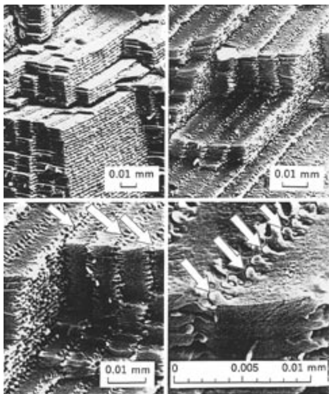
Imag. 3: Structura microscopică a cristalinului. Cele patru imagini mărite diferit cu ajutorul microscopului electronic arată structura strict ordonată a straturilor. Este redată comparativ și lungimea unei sutimi de mm. Prin articulații sferice unic realizate (indicate prin săgeți în cele două imagini de jos) straturile proteice sunt suturate într-o unitate elastică , astfel încât este posibilă realizarea distanțelor focale diferite prin modificarea formei cristalinului .
